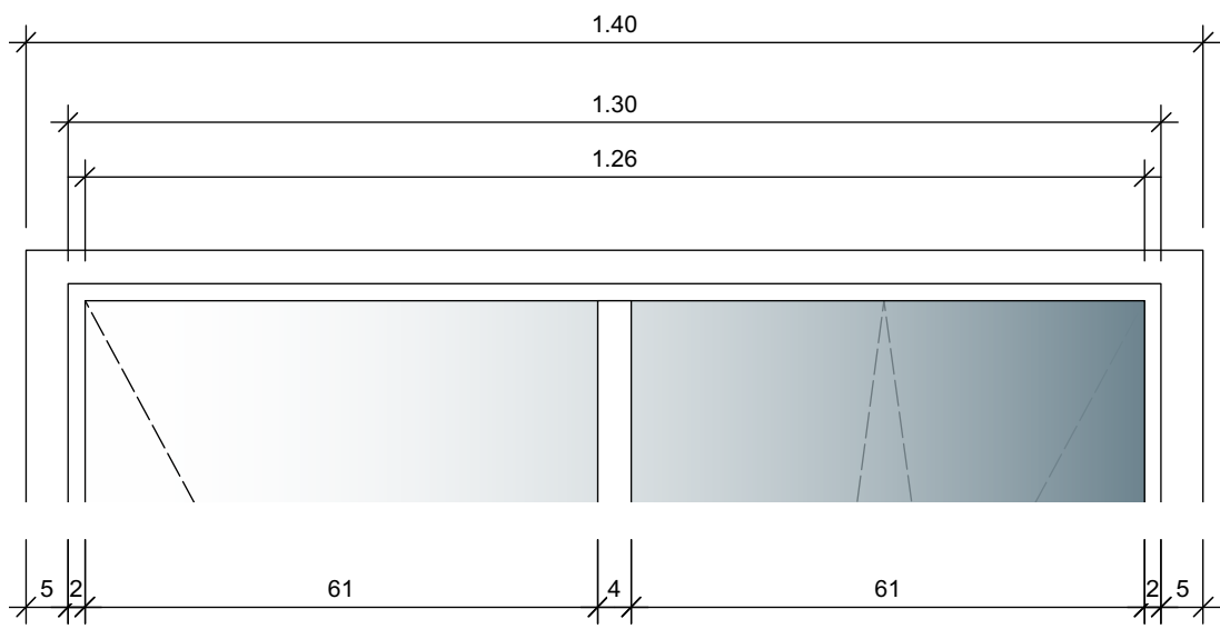
Ansicht M 1:10
