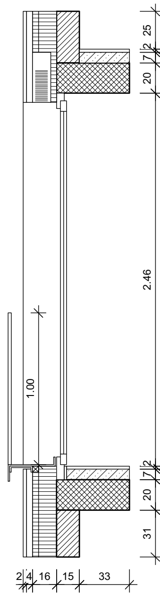
Schnitt M1:25
